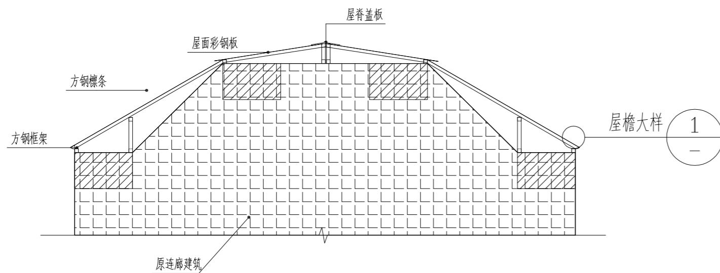
连廊加盖截面示意图 1:100
