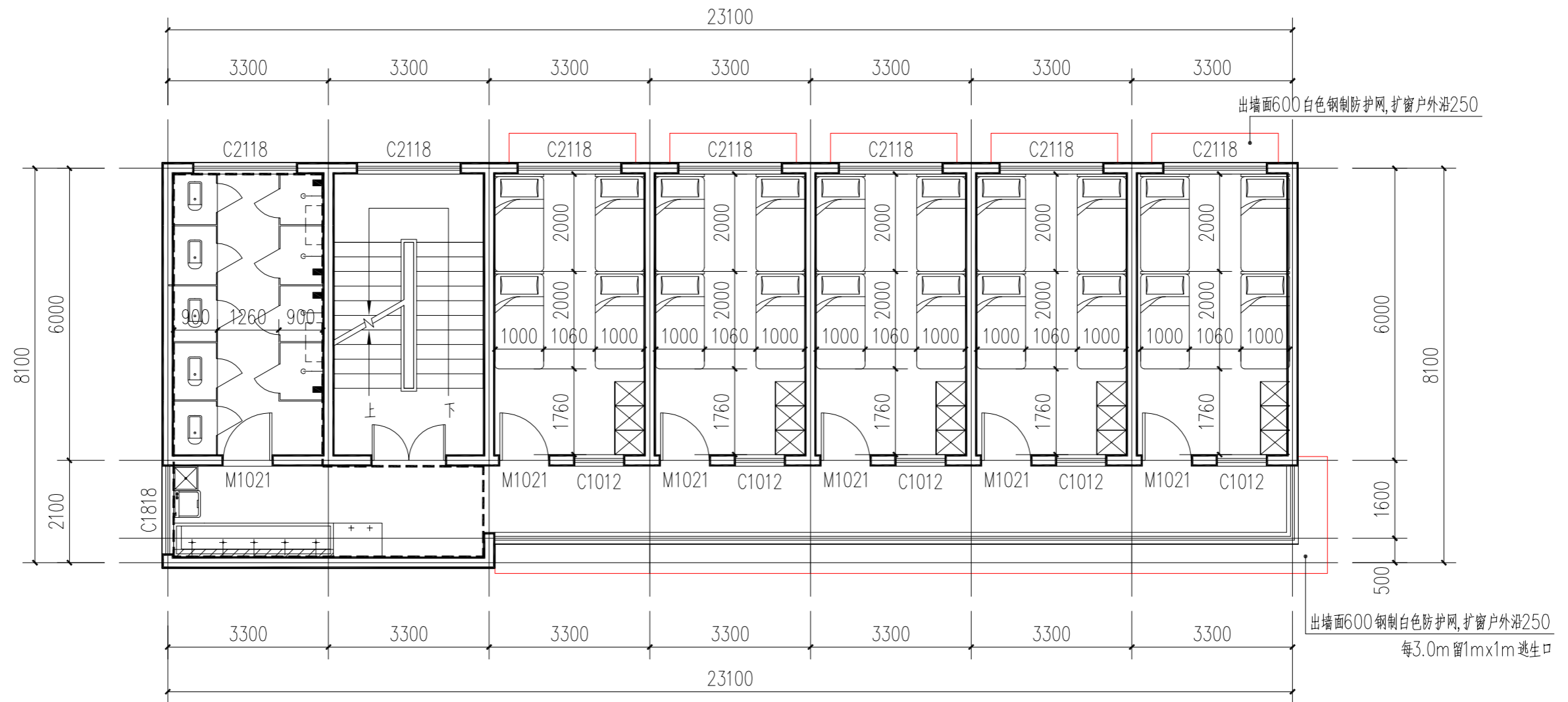
药剂楼4\6\7楼宿舍加防护网 1:100
