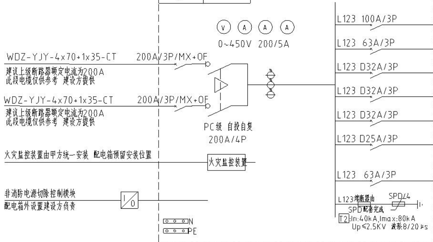
BAT1配电箱系统图
