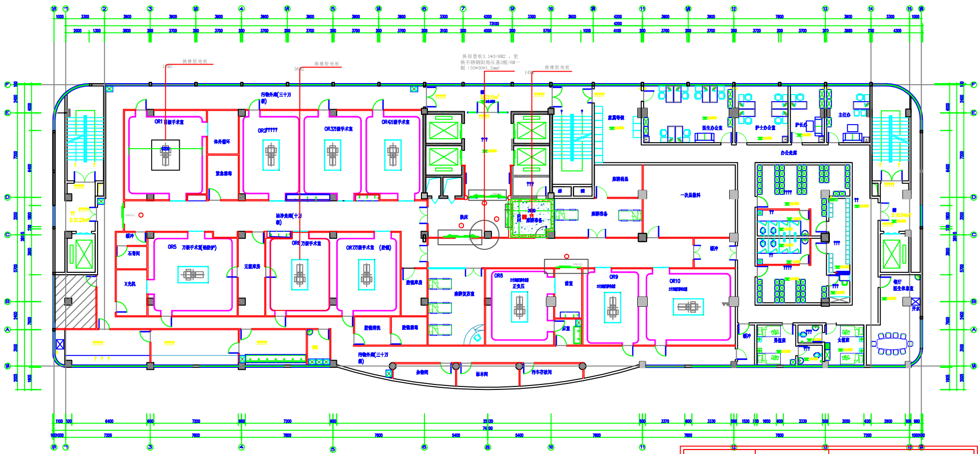
三层平面布置图 手术室 1:100
